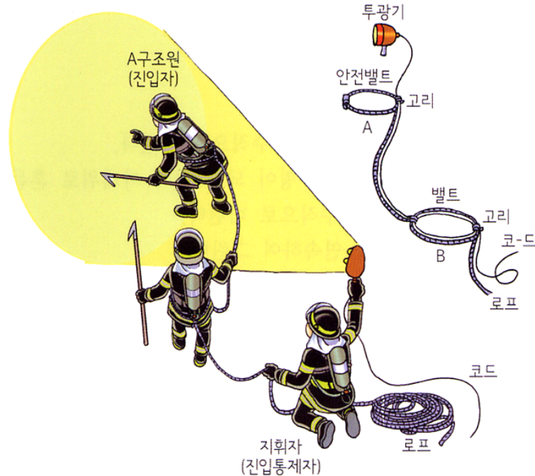
[그림 1-36] 안전 로프 결합 요령
